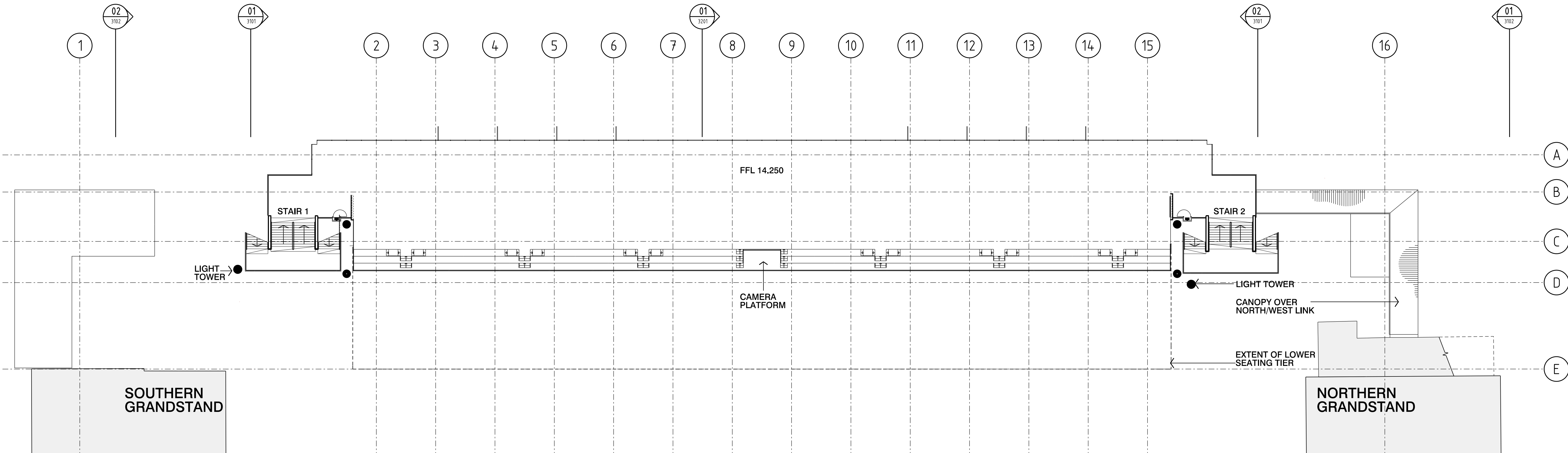
02 LEVEL 03 PLAN 1:250
