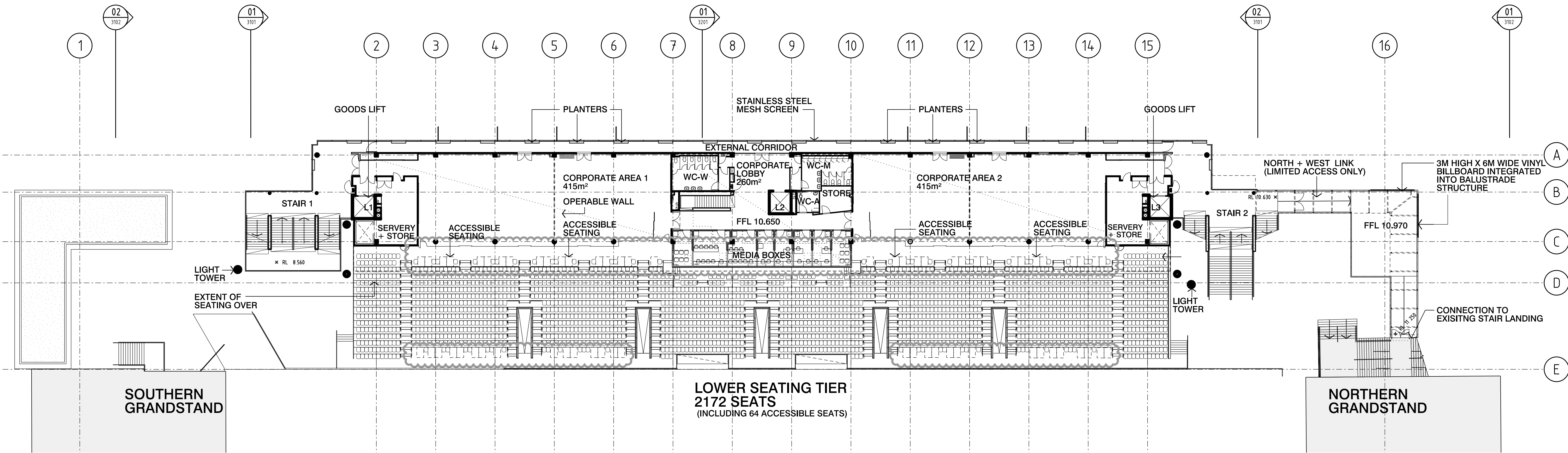
01 LEVEL 02 PLAN 1:250
